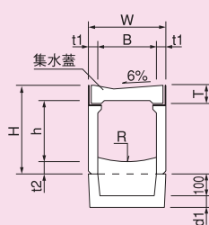
断面図
