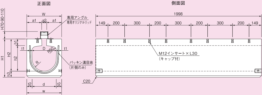
寸法表
