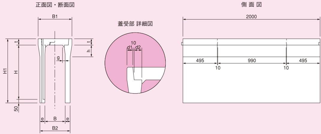
縦断用 (250型~600型)
