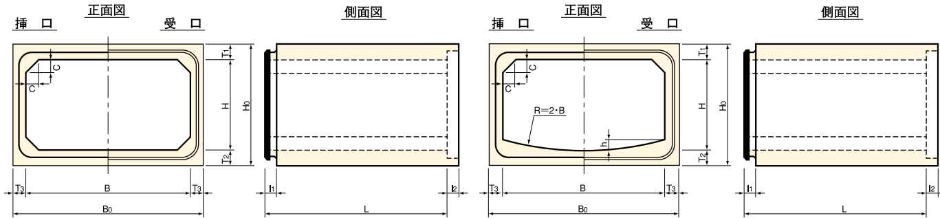
図1-1 ハンチタイプ
