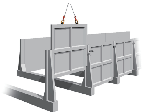
吊上げ状況：板
