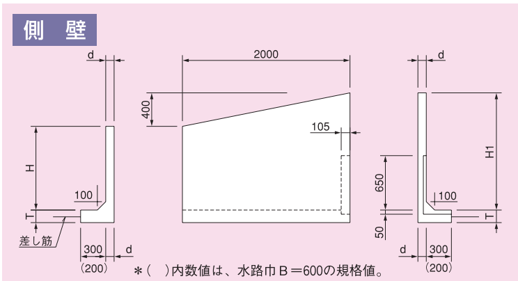
寸法表 (側壁)
