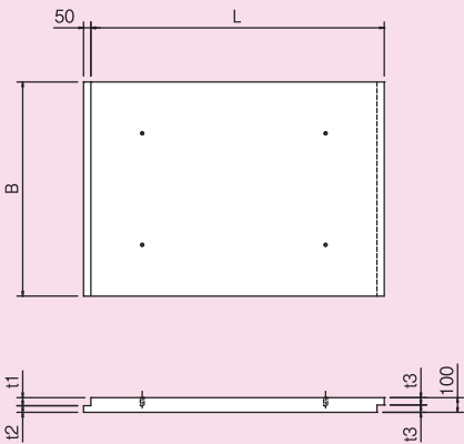
t=100mmタイプ
