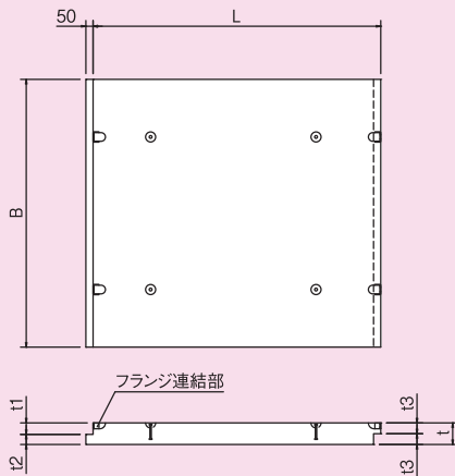
t=150・200mmタイプ
